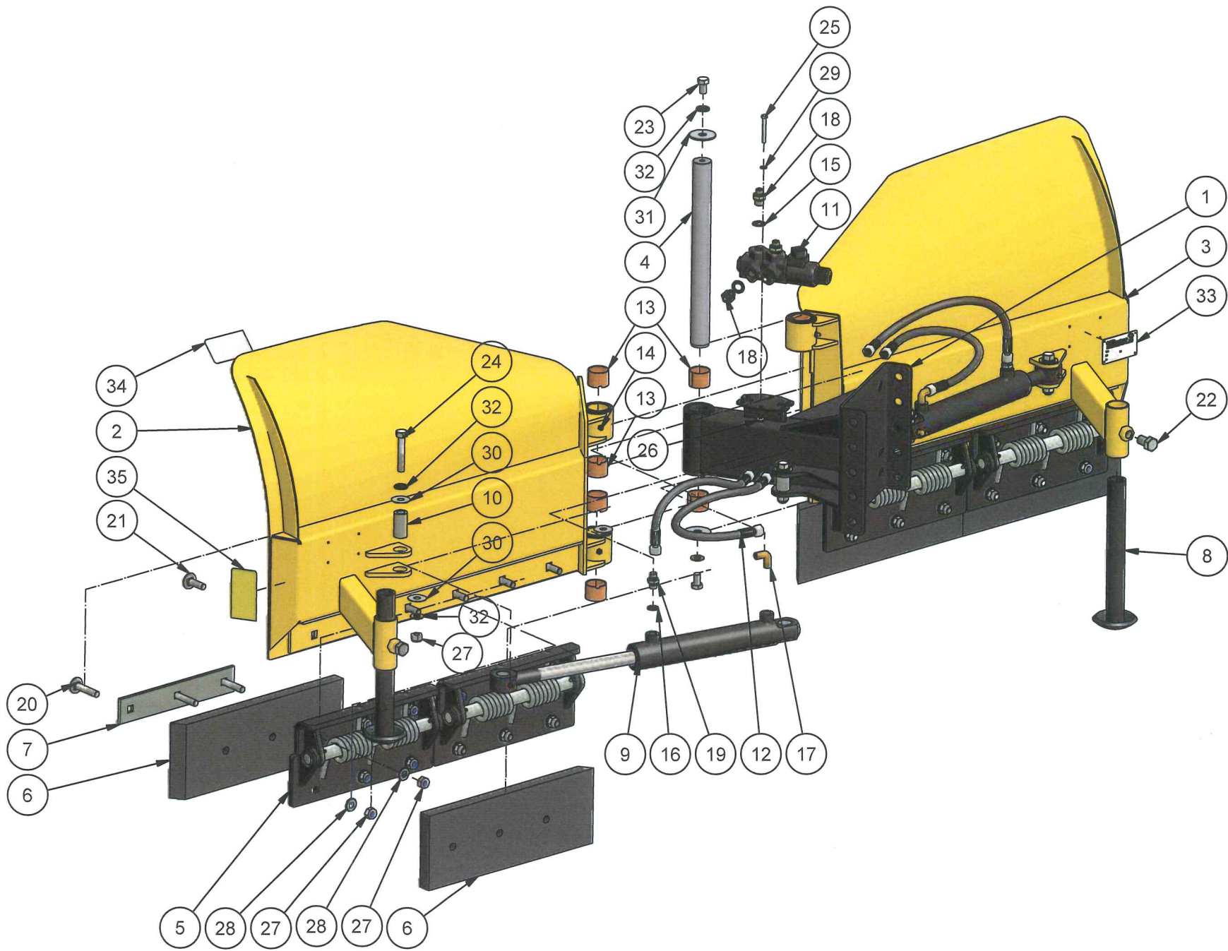
Sneskraber type PS 1300/1600 LK Model 2013 - med gummiskær
