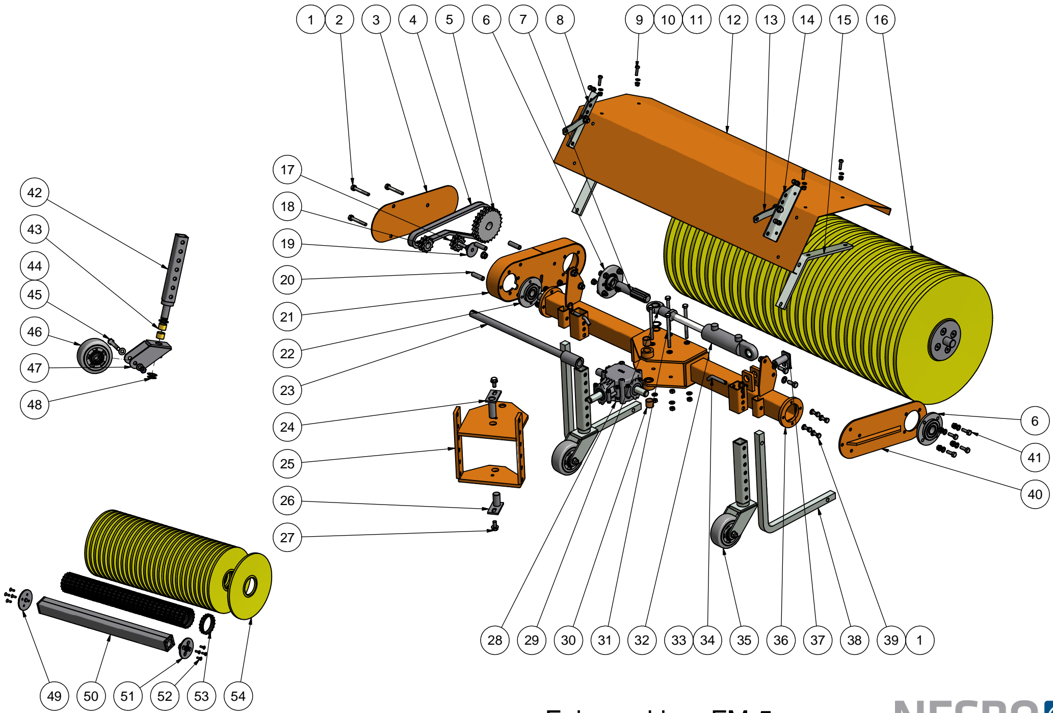
Fejemaskine FM-5
